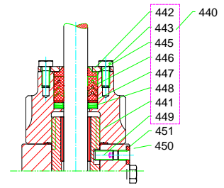
DN 20-100, PN 16-25
